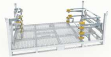
**Rack para transporte de assolho
