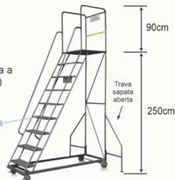
Degraus em Chapa Xadrez
